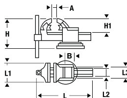
DRAAIBARE BANKSCHROEVEN
